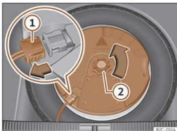
Fig. 206 En el maletero: desmontar el subwoofer.
